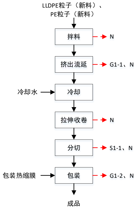
图 2-2 保鲜膜生产工艺流程图
