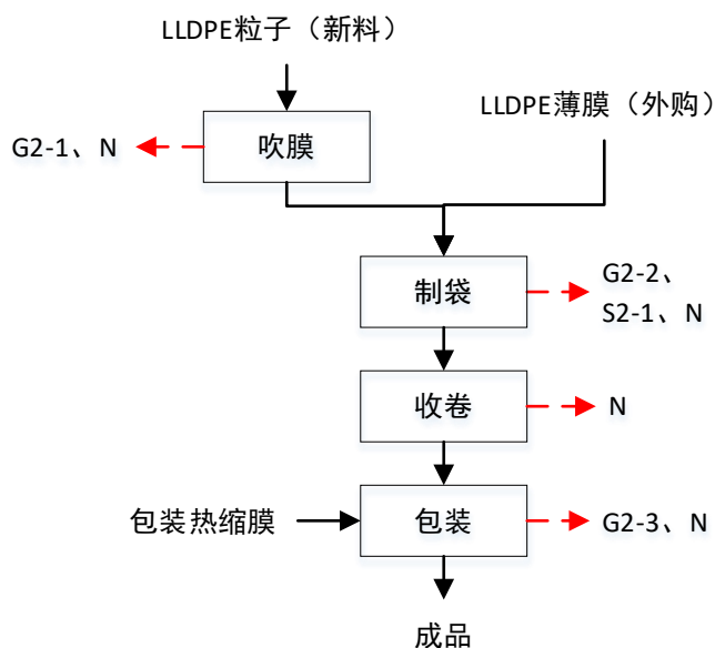
图 2-3 保鲜袋及垃圾袋生产工艺流程图 （注：Gn：废气污染物；Sn：固体废弃物；N：噪声）
