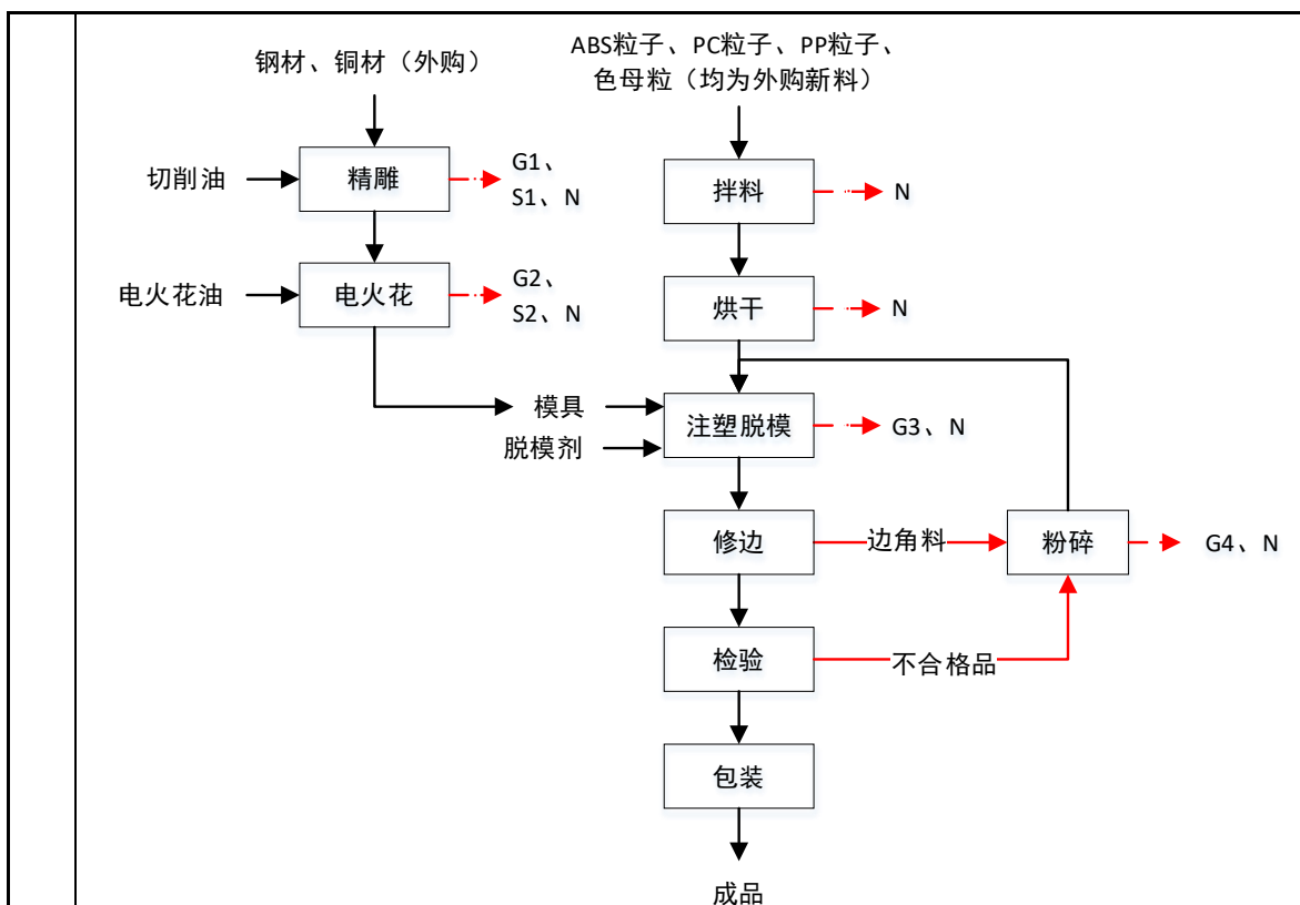
图 2-2 塑料玩具生产工艺流程图
